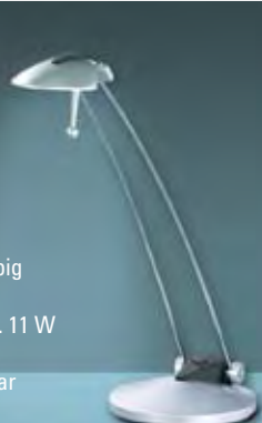
6574457.* Titanfarbig, EEK: C HAL 50 W, GY6,35, 2800 K, 850 lm H 535, B 160, T 160, D 150, A 500 mit Schalter € 49,00
