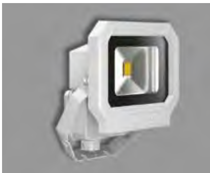
2615043.* Polycarbonat Weiß EEK: A+ 27 W, LED Platine austauschbar 3000 K, 2400 lm H 100, D 300 IP 65 € 188,00
